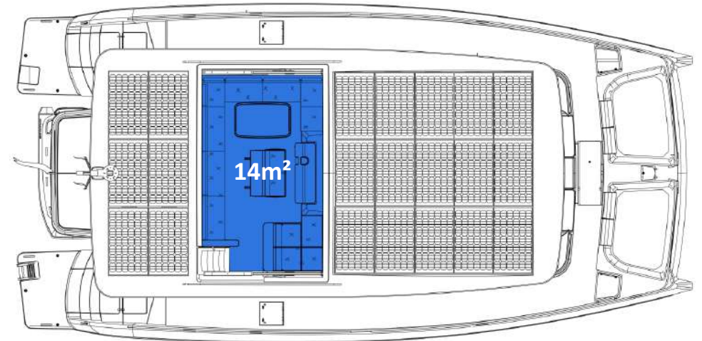
Flybridge
